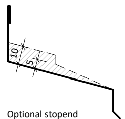
Optional stop end
